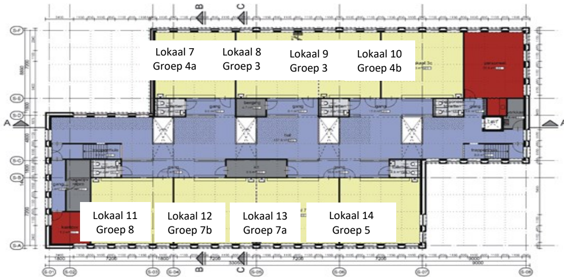
eerste verdieping 1:200
